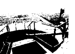
Zmodernizowany reaktor Biogradex I (widok z góry)
